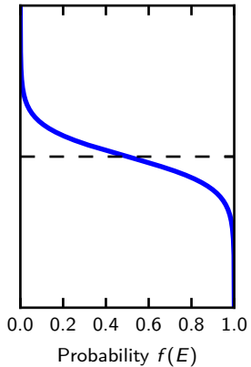
Fermi-Dirac Distribution
